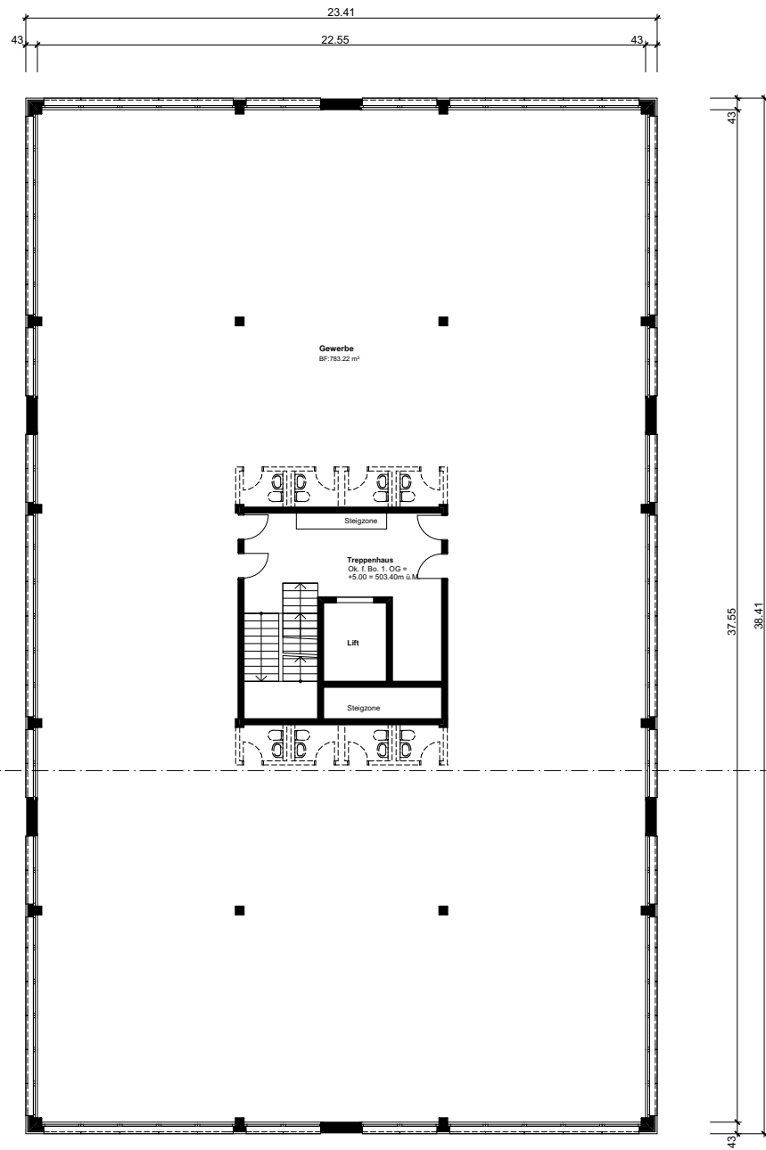
Grundriss 1. OG
