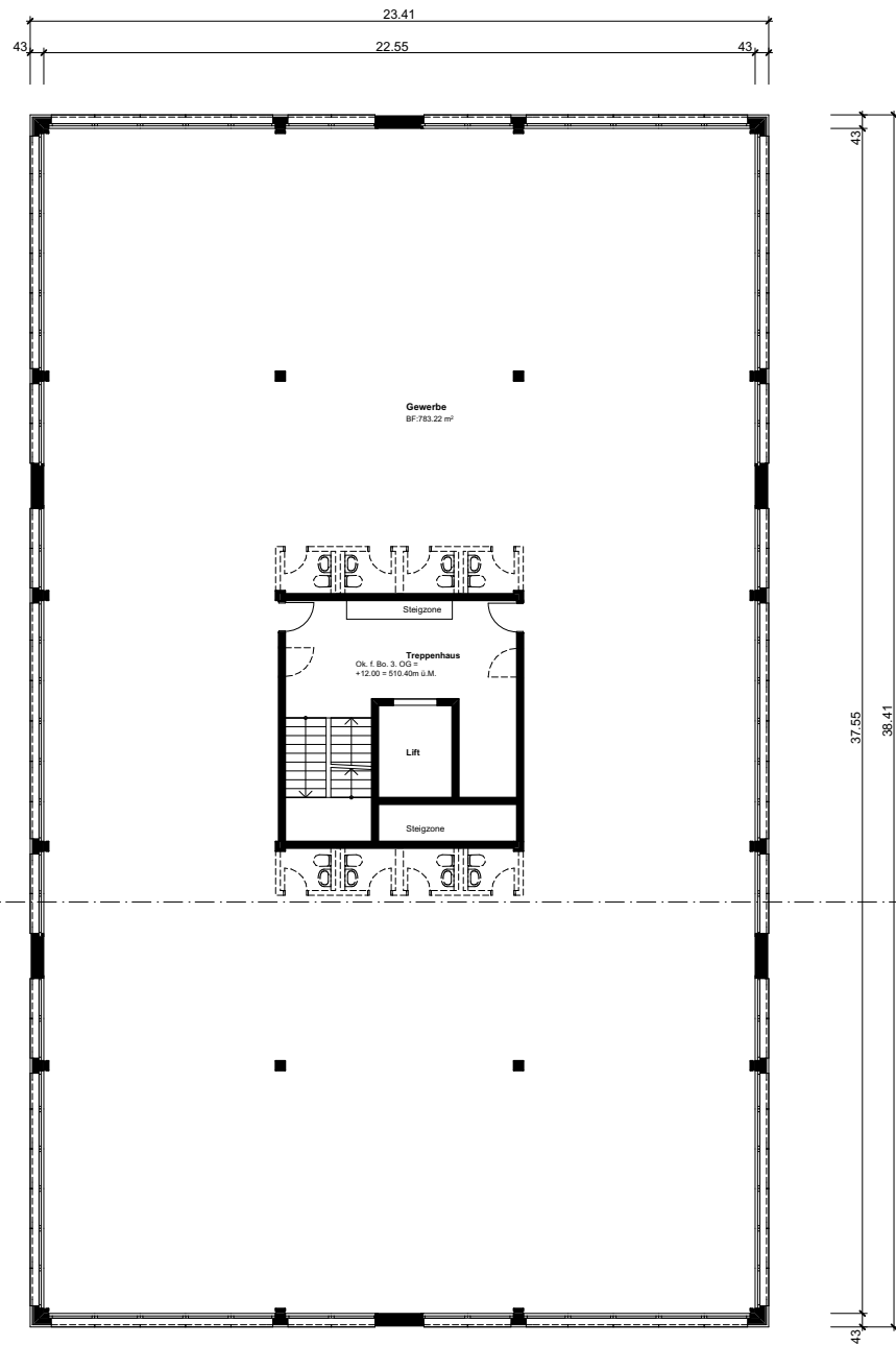
Grundriss 3. OG
