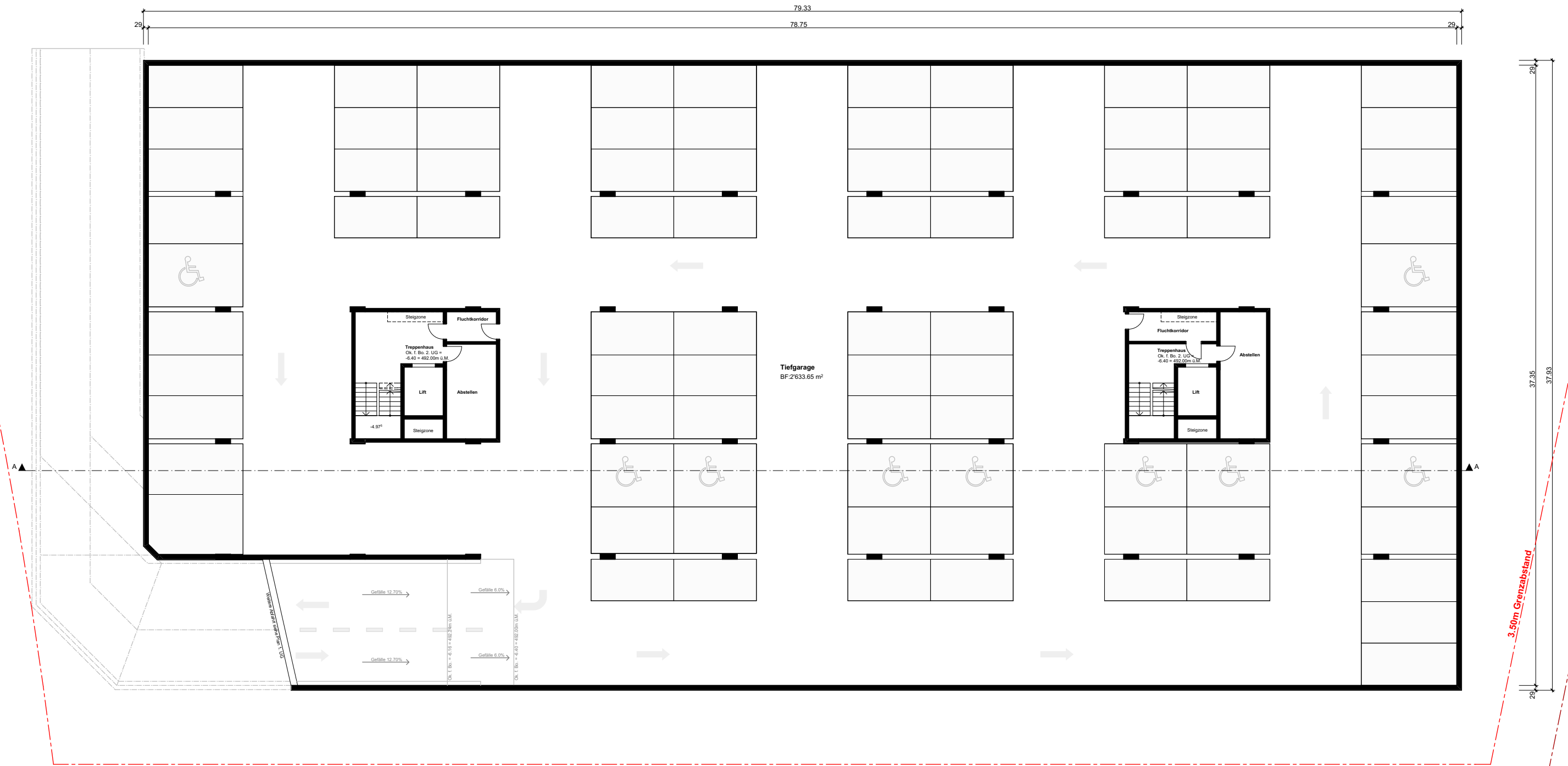
Grundriss 2. Untergeschoss
