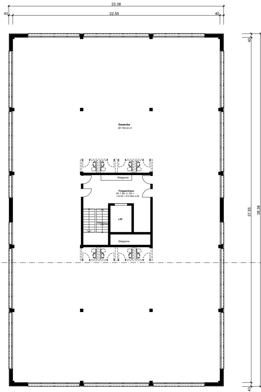
Grundriss 4. OG
