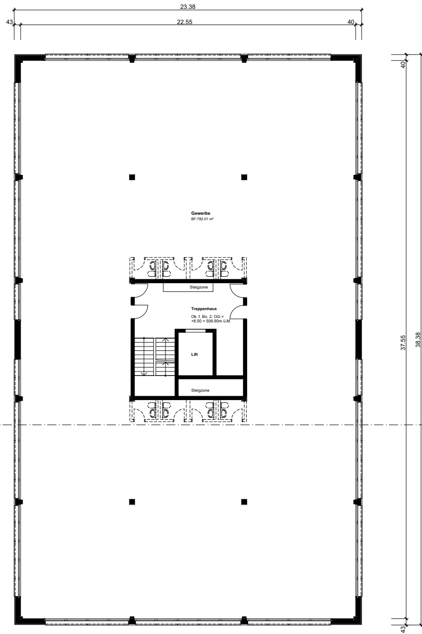
Grundriss 2. OG
