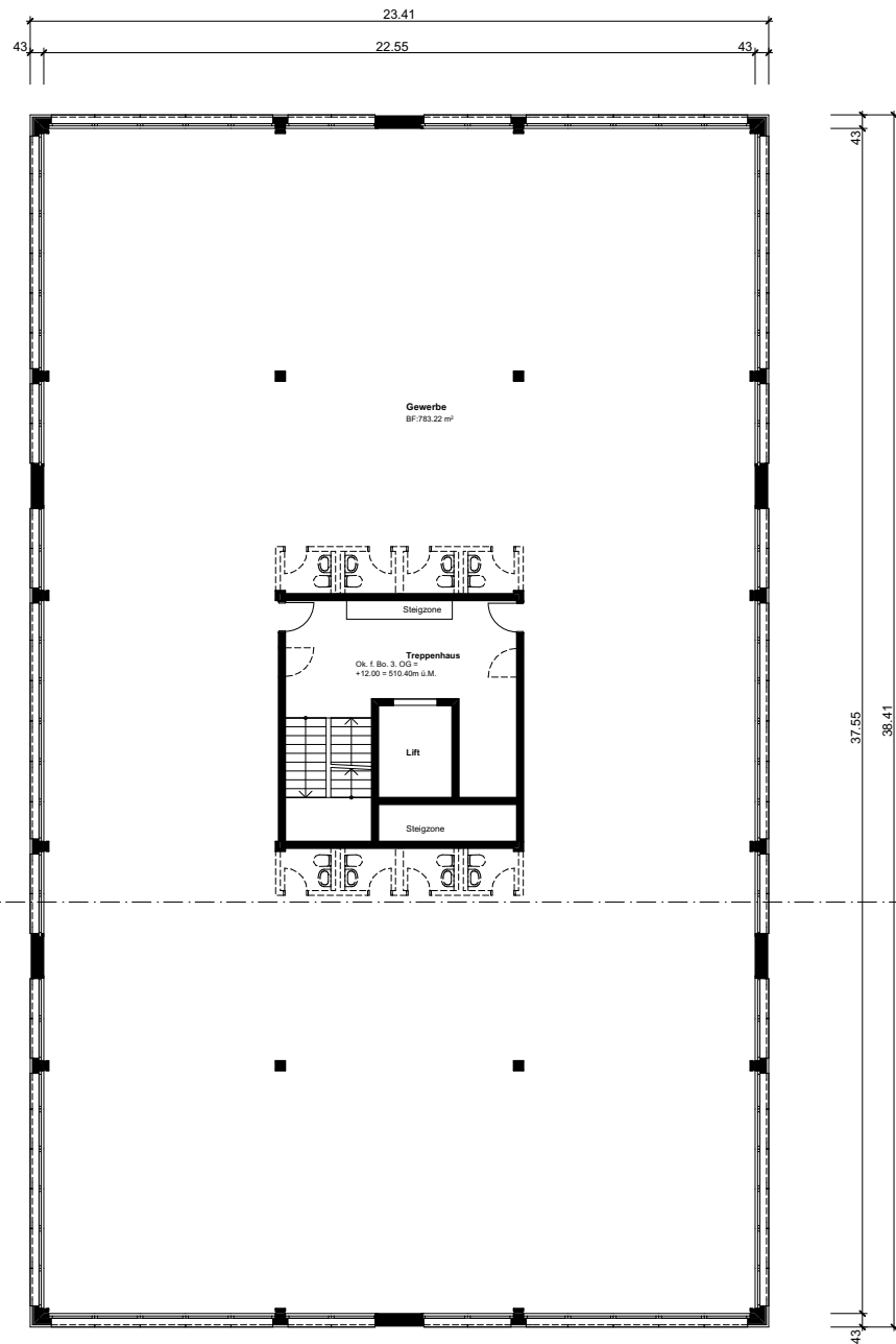
Grundriss 3. OG
