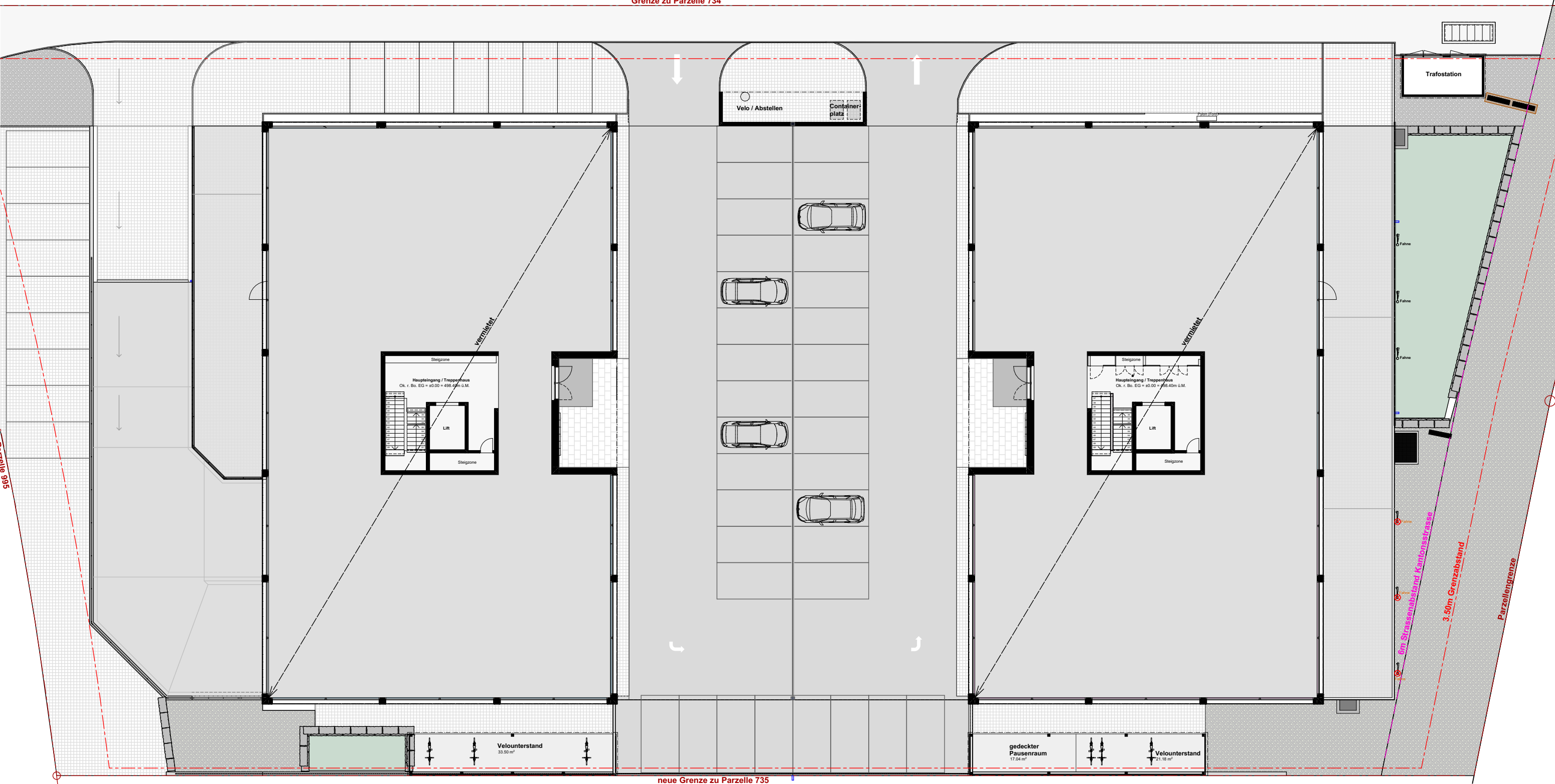
Grundriss Erdgeschoss Grenzstrasse 3a
